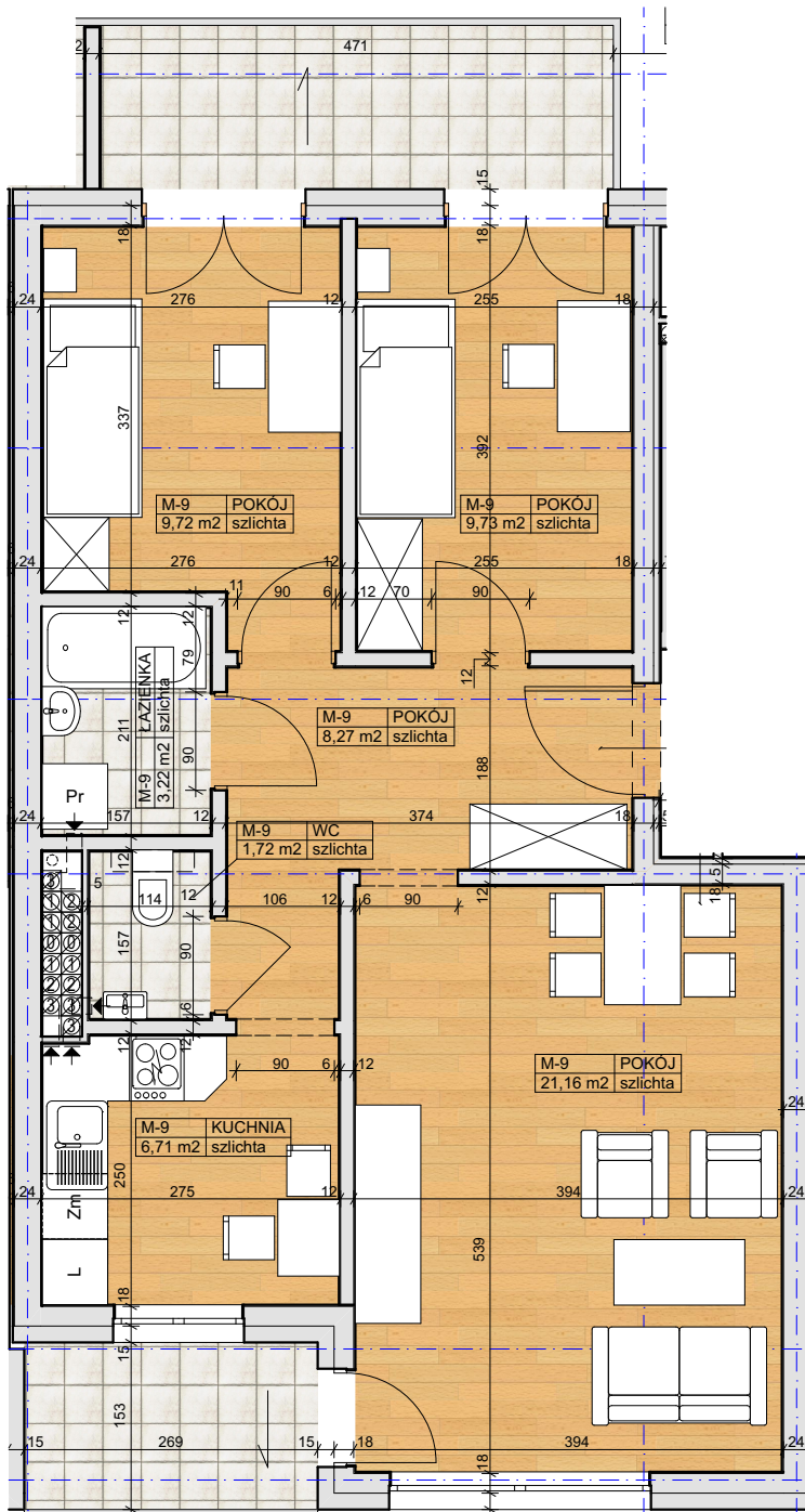
Rzut lokalu w skali 1:75
