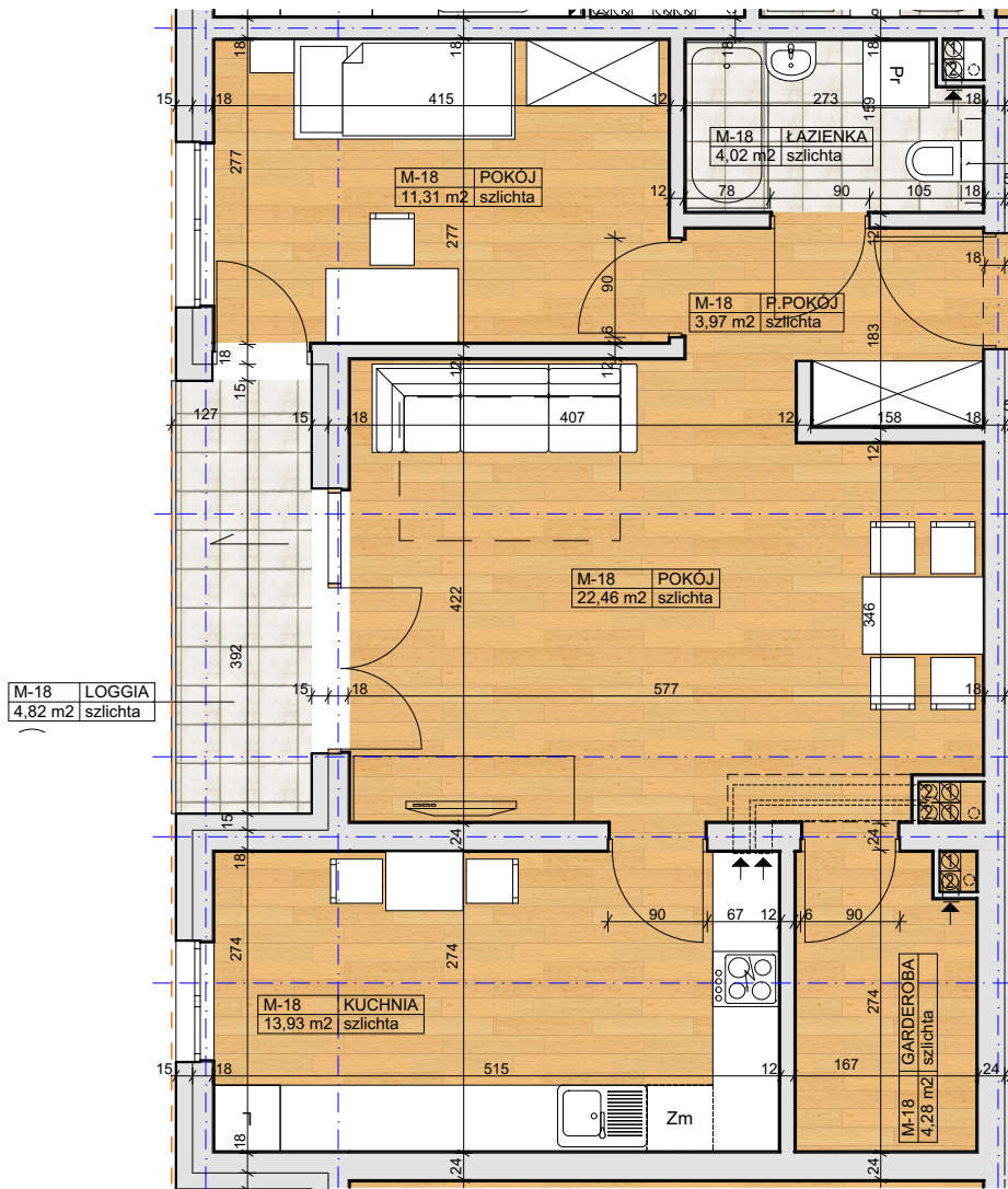
Rzut lokalu w skali 1:75
