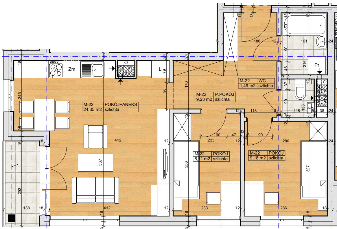
Rzut lokalu w skali 1:75
